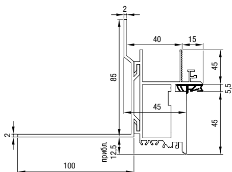
Оразмеряване на каса Zeroline
