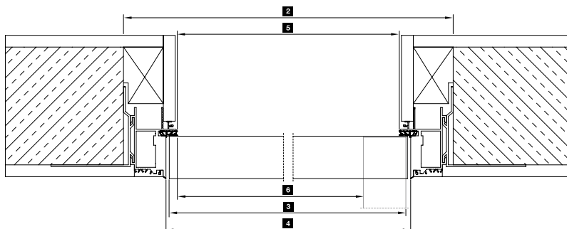
Хоризонтален разрез с платно без фалц
