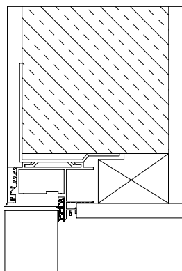
Хоризонтален разрез с врата без фалц
