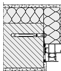
Karpleng Ankurpaigaldus
