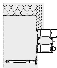
Karpleng Ankurpaigaldus
