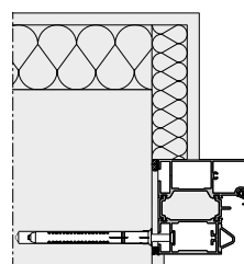
Karpleng Tüübelpaigaldus
